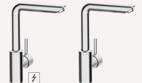
Einhebelmischer für Spültisch, seitenbedient, mit Pinhebel , schwenkbarer Auslauf, Höhe: 276 mm, Ausladung: 164 mm
